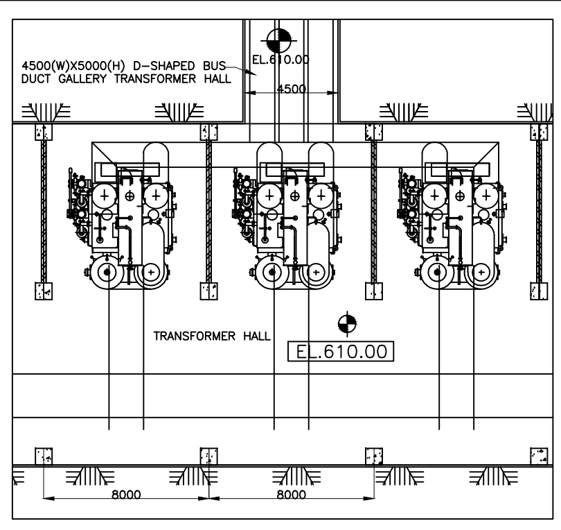
DETAIL-B
